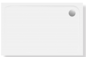
DIANA Plus2 Acryl-Rechteck-Brausewanne superflach, Tiefe 35 mm, Ablaufloch 90 mm, weiß, 900 x 750 mm, (MB224101001) 208,10 € 900 x 800 mm, (MB224102001) 208,10 € 1000 x 800 mm, (MB224105001) 229,80 € 1200 x 800 mm, (MB224106001) 276,10 € 1200 x 900 mm, (MB224107001) 297,50 € 1400 x 900 mm, (MB224108001) 323,80 €
